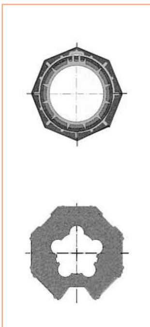
■ adattatore DOPPIA CORONA per tubo OTTAGONALE diametro 70
