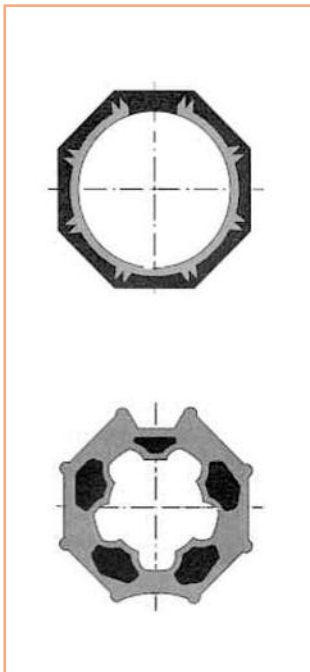
■ Adattatore CORONA per tubo OTTAGONALE diametro 60
